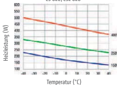
Heizleistung-/Umgebungstemperatur-Diagramm CS 028/CSL 028
