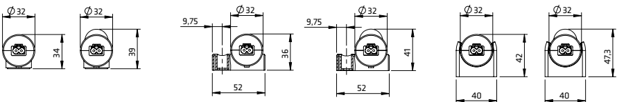
Seitenansicht Magnetbefestigung
